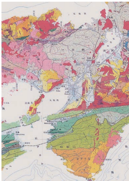
近畿地域の地質図 赤い部分が火成岩
